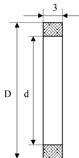
Рисунок 2.13 Уплотнительное кольцо для фланцевого соединения.
