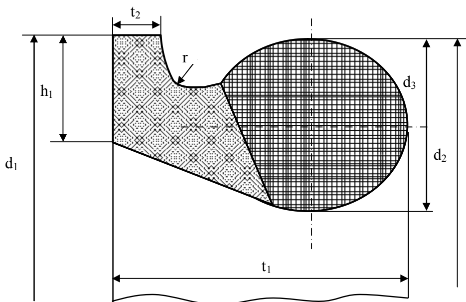
Рисунок 2.3 Уплотнительное резиновое кольцо под соединение «Тyton».
