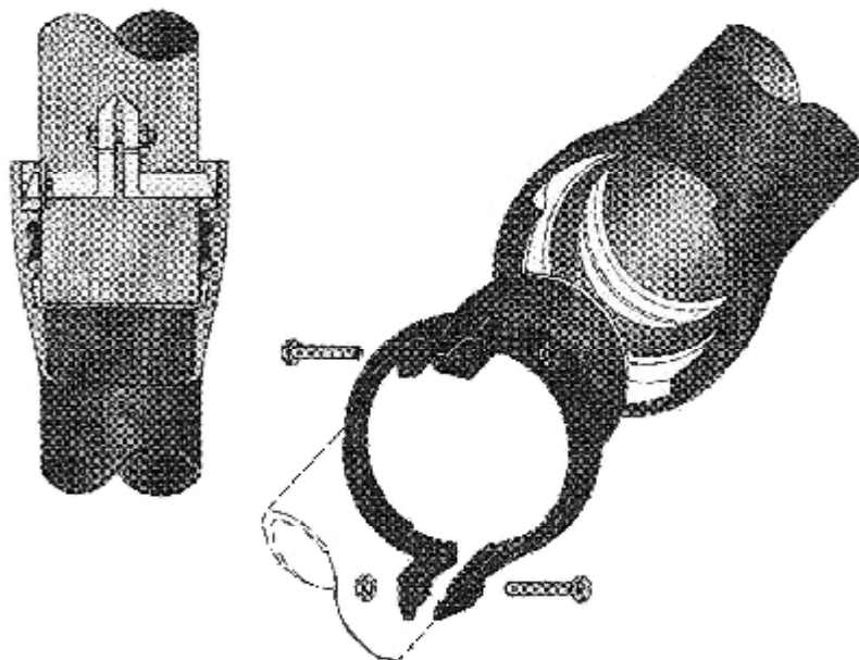
Рисунок 6.10 Специальное приспособление – стяжные кольца, заменяющее наплавленный валик.
