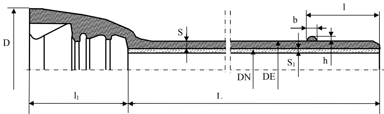
Рисунок 2.5 Труба раструбная под соединение «RJ».
